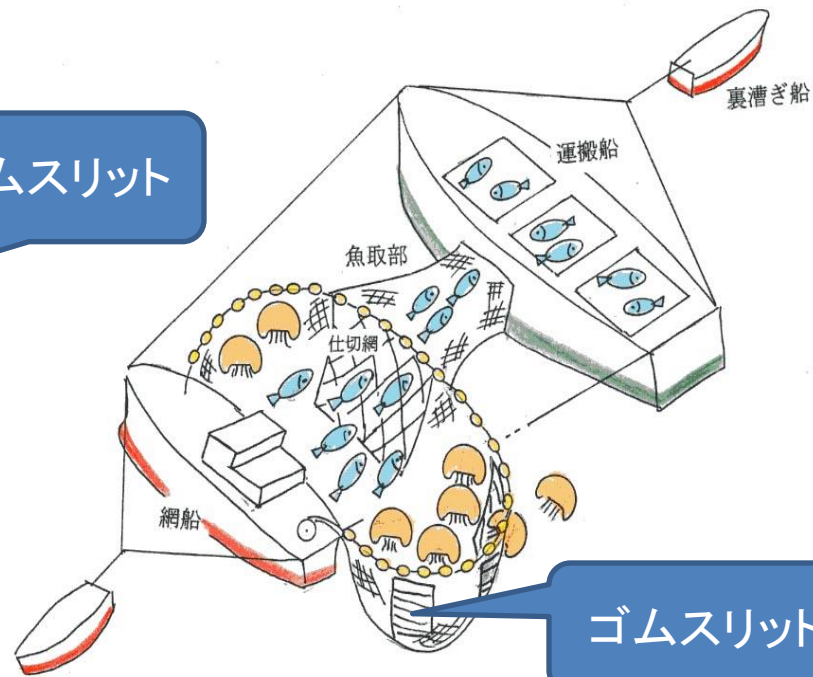
裏漕ぎ船 大型クガ防除網 仕切網 使用時概要図
