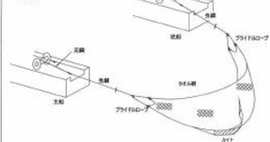
4. 曳網
