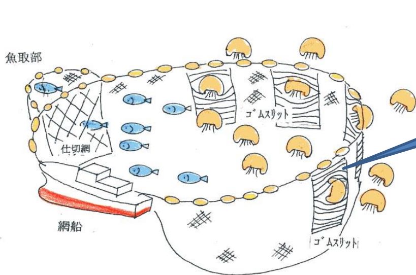
大型クガ防除網 ゴムスリット 使用時概要図
